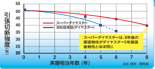
■物性変化(耐候性促進試験)
