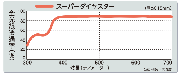
■光線透過特性
